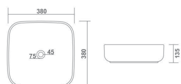
ETIOS L 380 W 380 H 135 mm 15" x 15"
