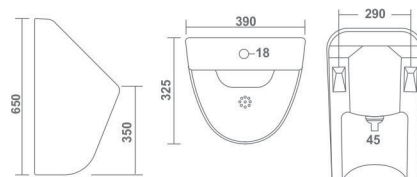
BARCA L 390 W 325 H 650 mm
