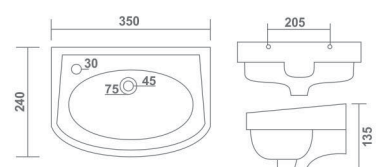
MINT L 350 W 240 H 135 mm 14" x 10"
