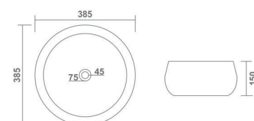
MOON L 385 W 385 H 150 mm 15" x 15"
