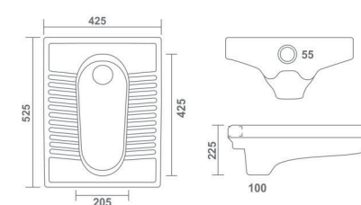
ORISSA PAN - 21" L 525 W 425 H 225 mm
